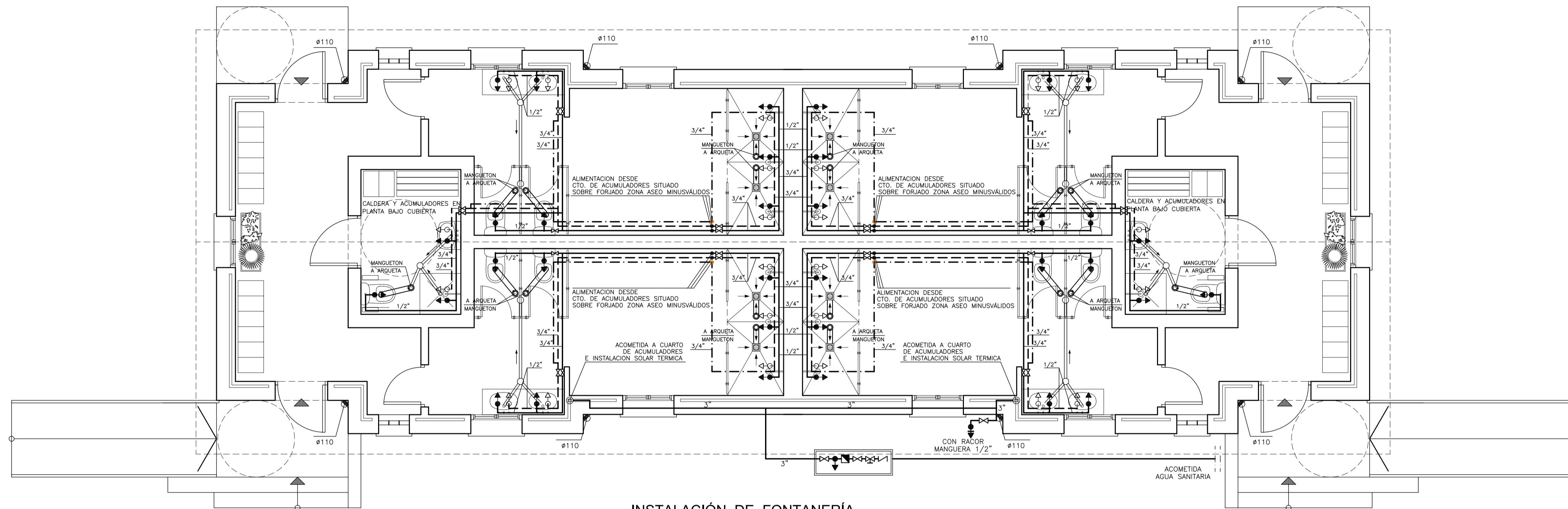
INSTALACIÓN DE FONTANERÍA ESCALA 1/50
