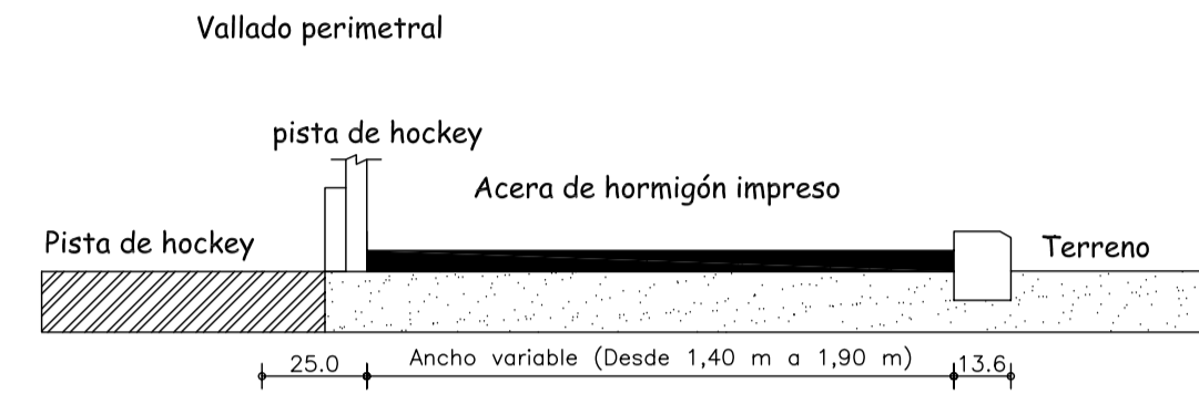
SECCIÓN TIPO ACERA PERIMETRAL E 1/20
