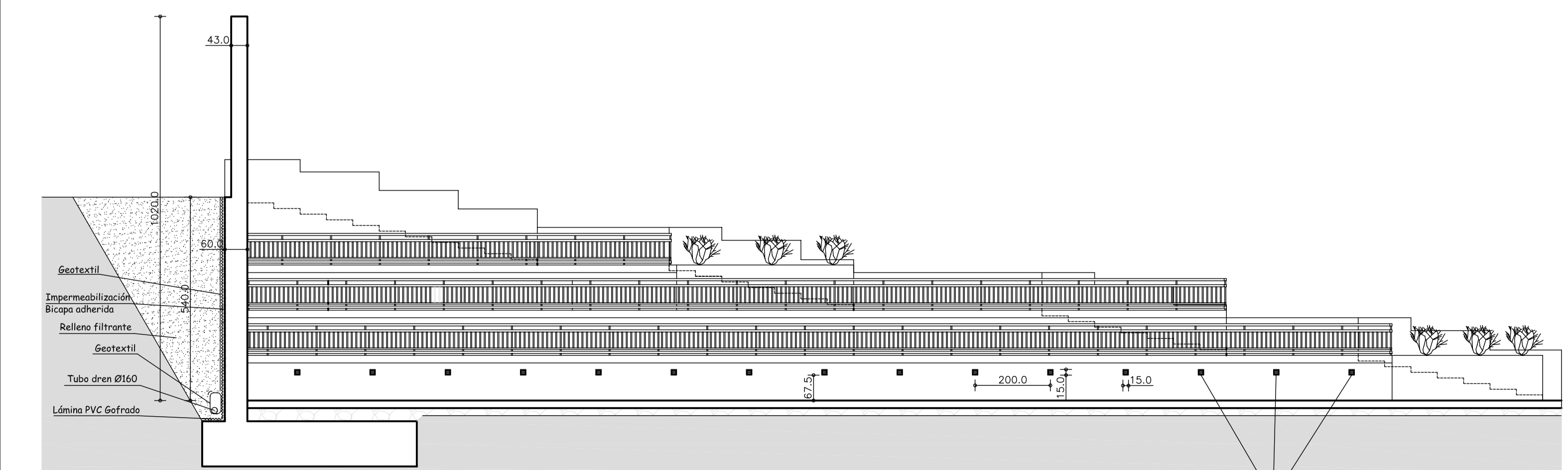
GRADAS DEL FRONTÓN SECCIÓN B-B' E 1/100
