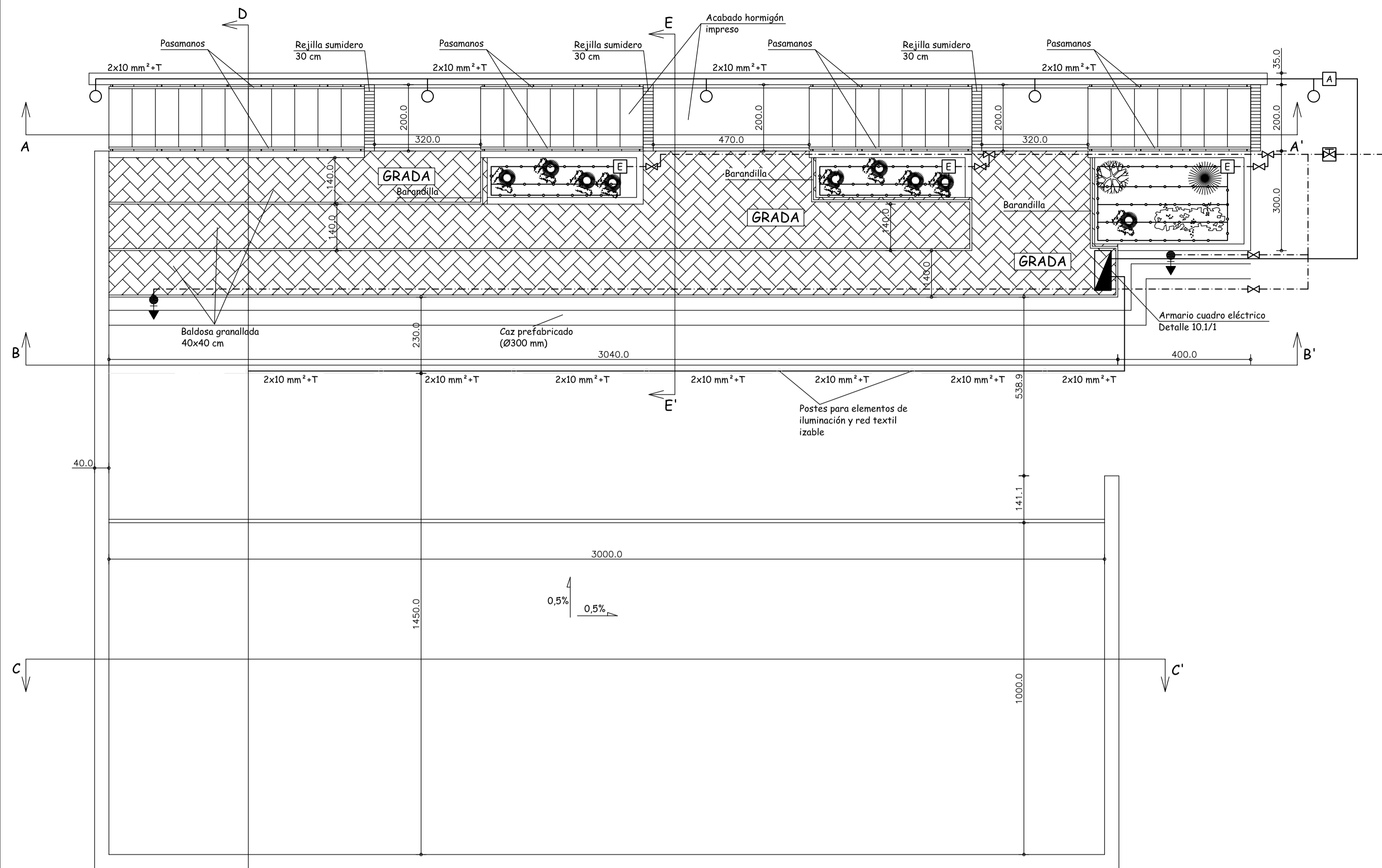
FRONTÓN. COTAS. INSTALACIÓN ILUMINACIÓN/FONTANERÍA/RIEGO PLANTA E 1/100
