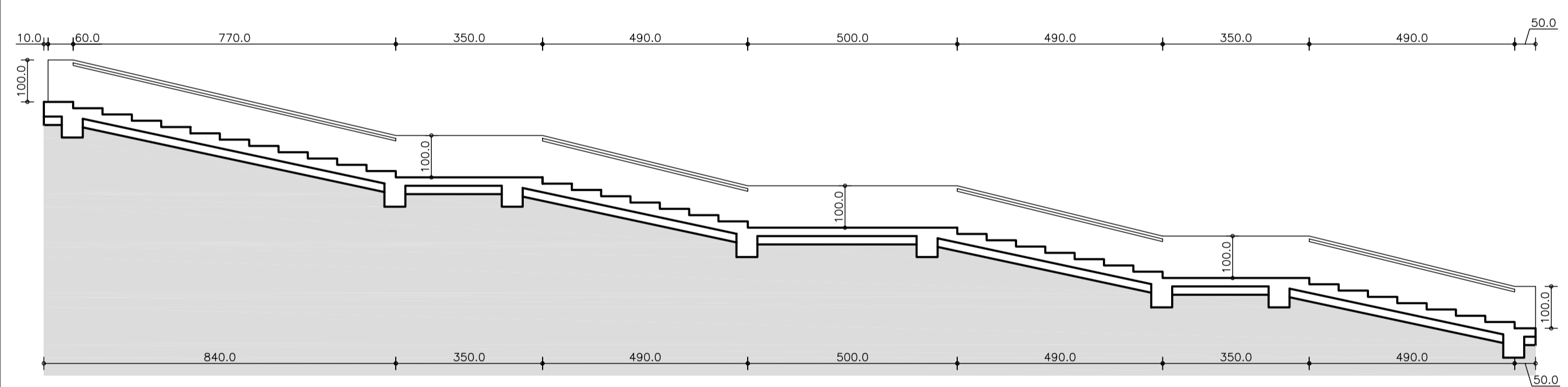
GRADAS DEL FRONTÓN SECCIÓN A-A' E 1/100
