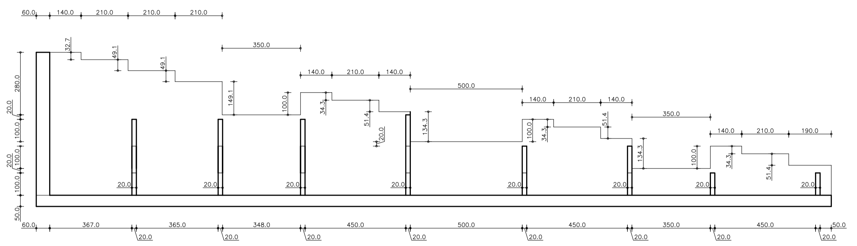
FRONTÓN. COSTILLAS GRADAS ALZADO E 1/100
